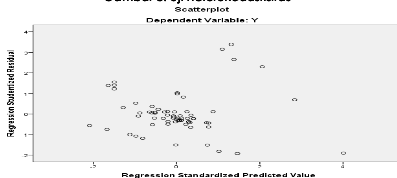
Gambar 3. Uji Heteroskedastisitas
